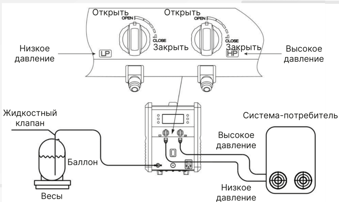
Схема станции
